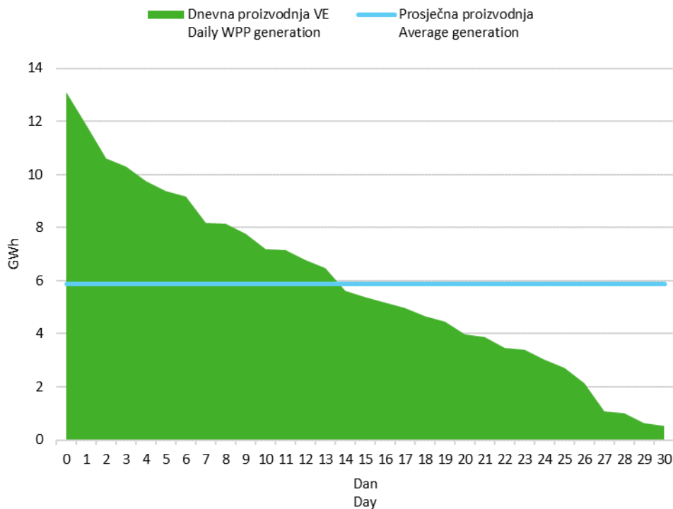
Slika 6 Krivulja trajanja dnevne proizvodnje vjetroelektrana u svibnju 2020. godine
