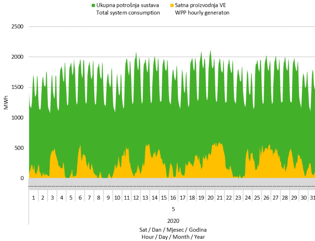
Slika 7 Usporedba satnog dijagrama opterećenja sustava i proizvodnje vjetroelektrana u svibnju 2020. godine
