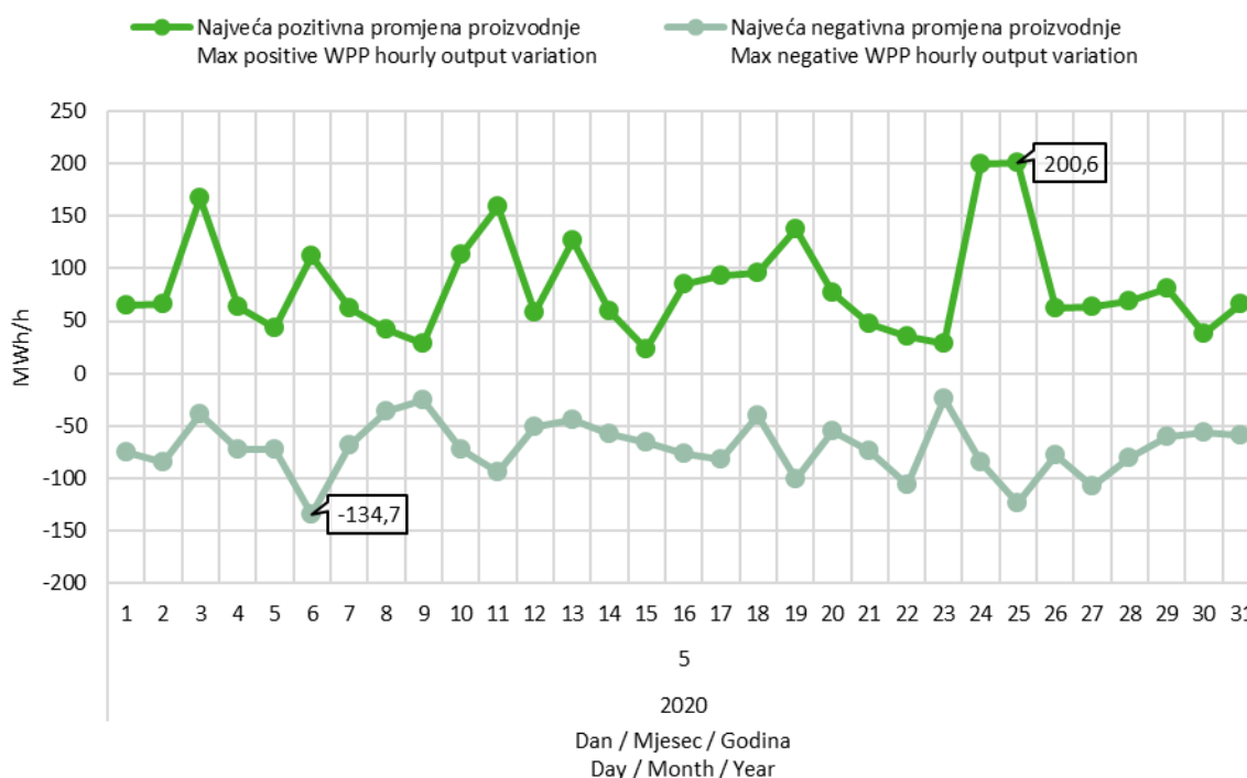
Slika 9 Maksimalna pozitivna i maksimalna negativna promjena satne proizvodnje VE u svibnju 2020. godine
