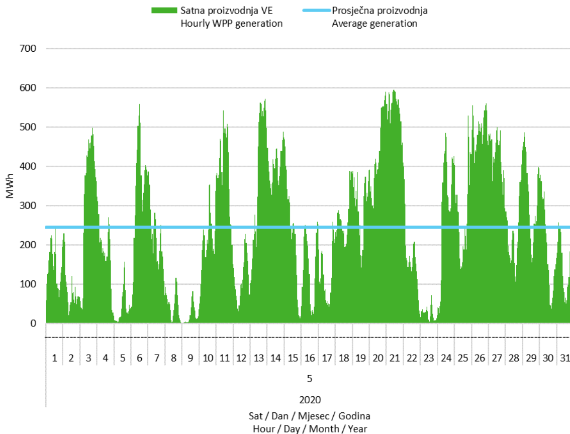
Slika 2 Satna proizvodnja svih vjetroelektrana u svibnju 2020. godine
