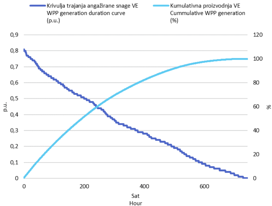
Slika 3 Krivulja trajanja angažirane snage svih VE i kumulativna proizvodnja VE u svibnju 2020. godine u jediničnim vrijednostima
