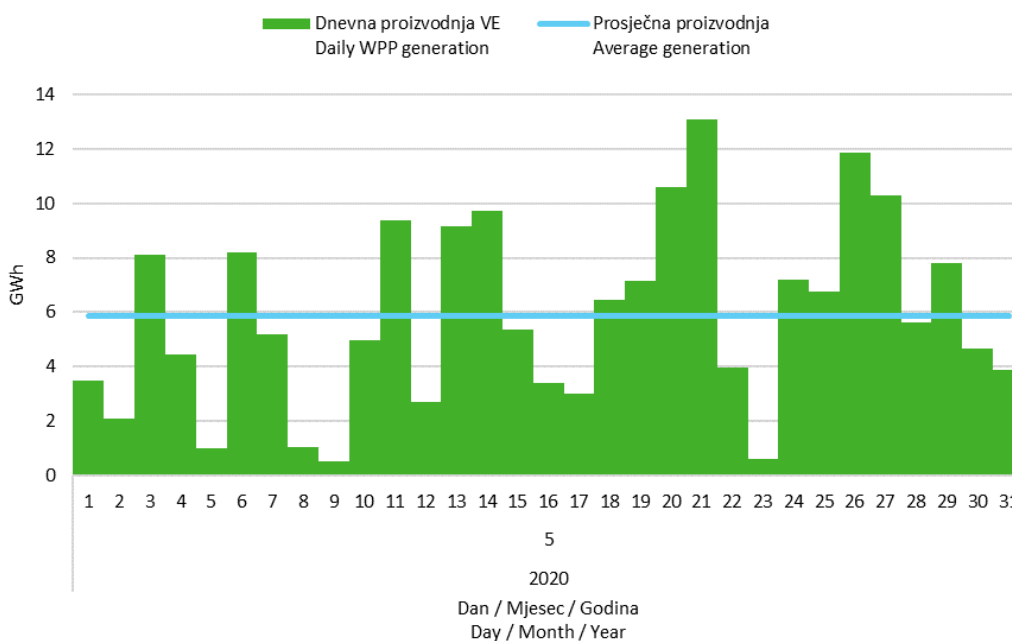
Slika 5 Dnevna proizvodnja svih vjetroelektrana u svibnju 2020. godine
