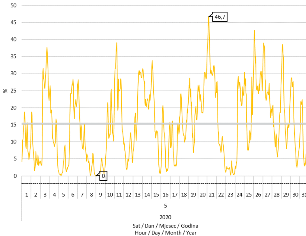
Slika 8 Udio proizvodnje vjetroelektrana u pokrivanju satnog opterećenja elektroenergetskog sustava u svibnju 2020. godine
