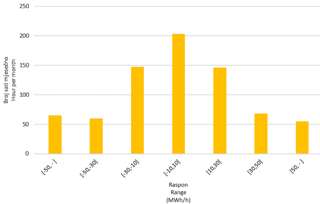
Slika 10 Statistička raspodjela satnih promjena proizvodnje VE u svibnju 2020. godine
